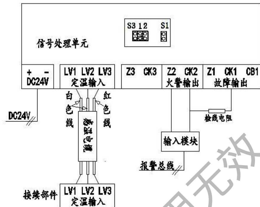
图 4 探测器应用系统图
